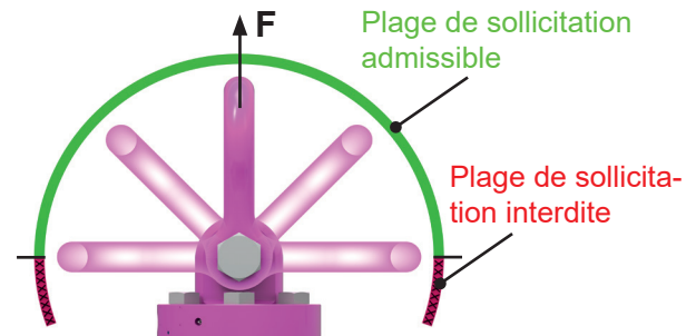
Fig. 5 : Inclinaison vers le sens dans lequel l'anneau se rabat (vert = plage de sollicitation admissible)
