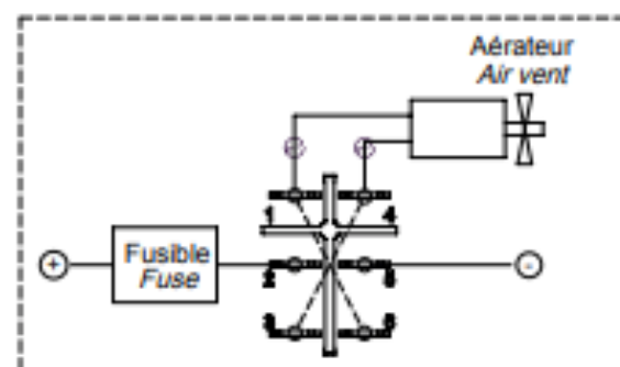
Schéma de branchement / Connection diagramme
